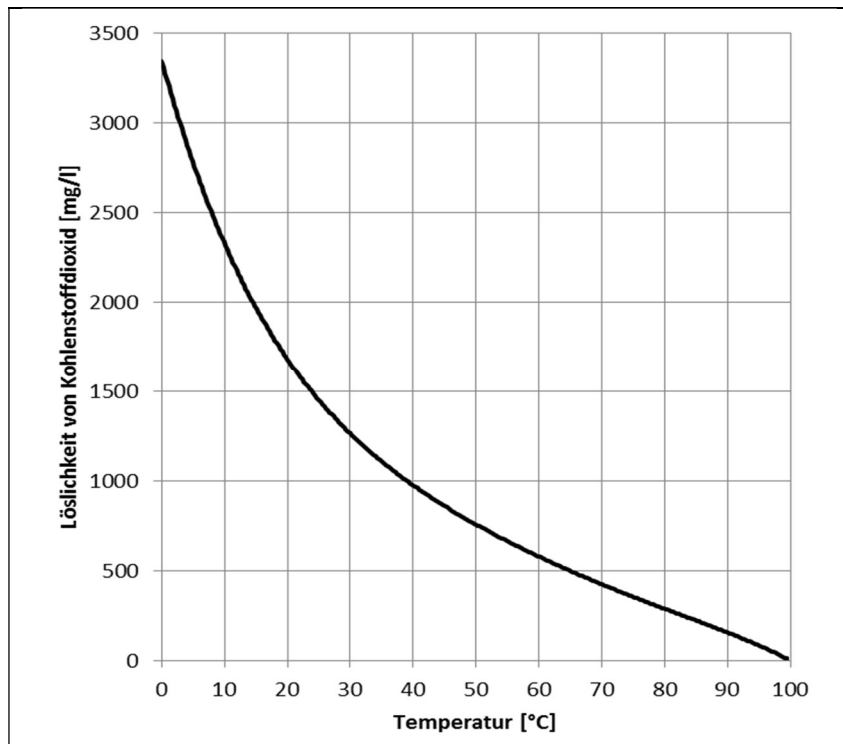
Diagramm: Löslichkeit von Kohlenstoffdioxid in salzfreiem Wasser in Abhängigkeit von der Temperatur unter Atmosphärendruck
