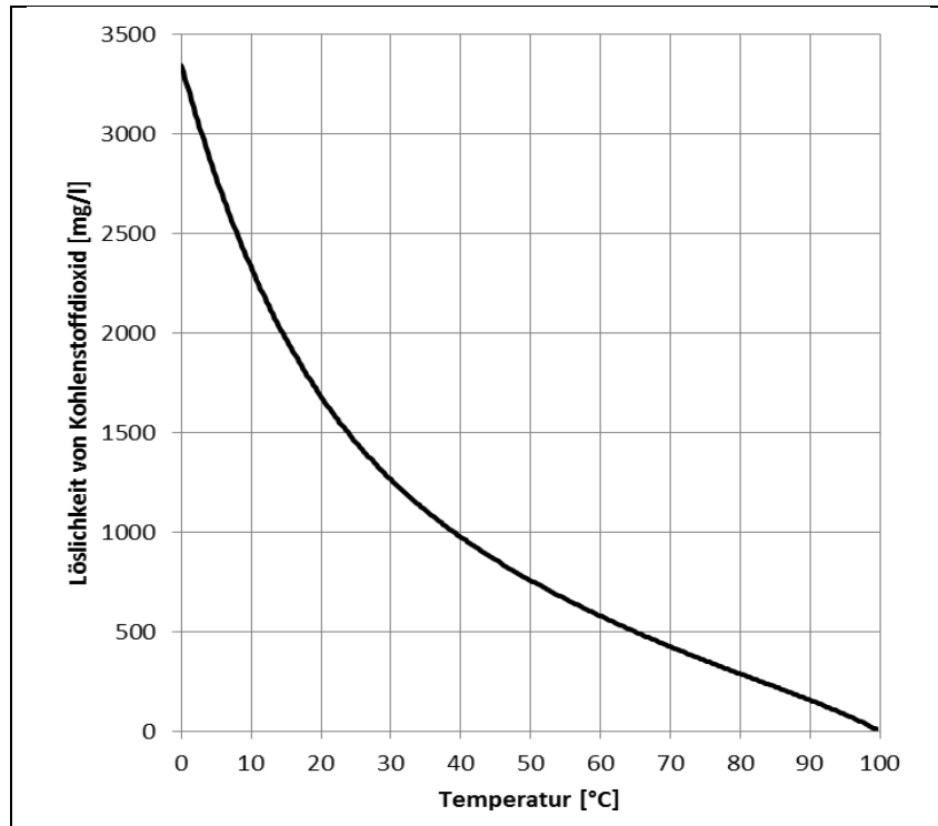
Diagramm: Löslichkeit von Kohlenstoffdioxid in salzfreiem Wasser in Abhängigkeit von der Temperatur unter Atmosphärendruck
